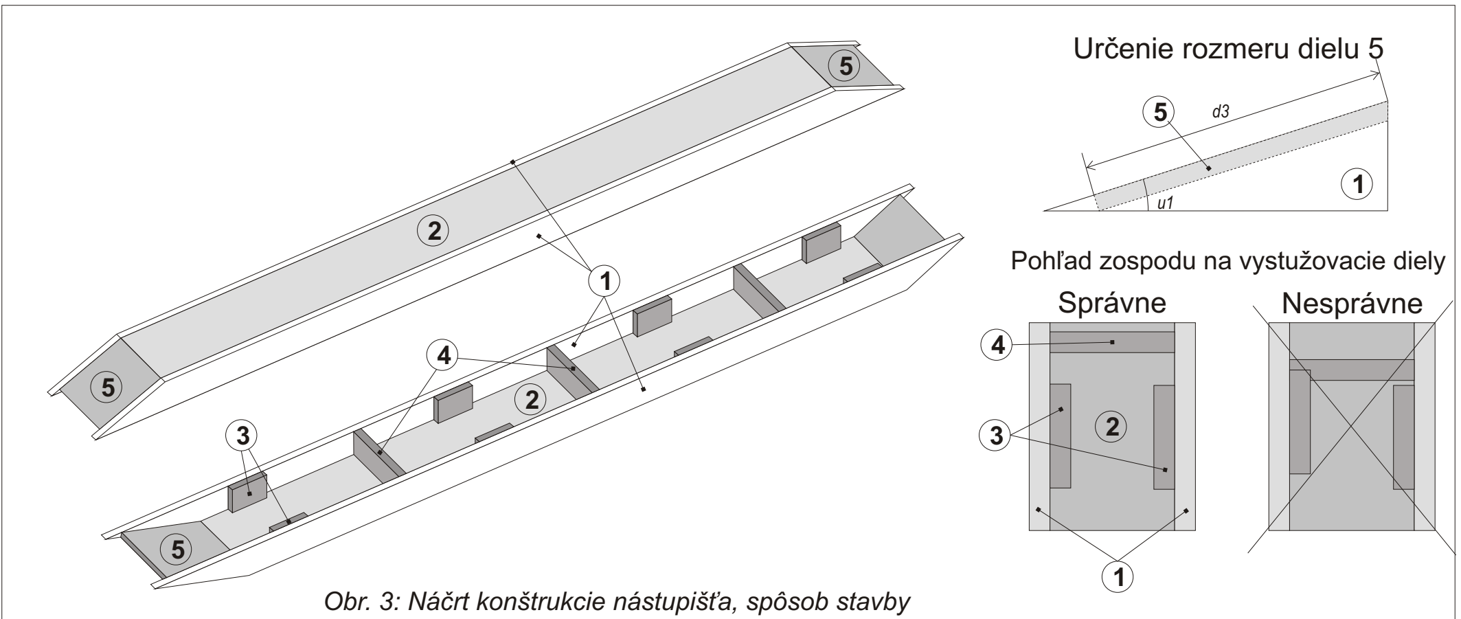
Obr. 2 : Diely ná výrobu nástupišťa
